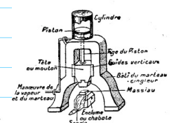
Fig. 52. — Marteau-pilon.
