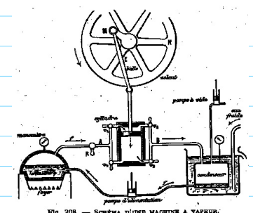
Fig. 208. — SCHEMA D'UNE MACHINE A VAPEUR.
