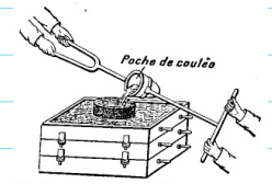
Fig. 73. — Moulage par coulée « en descente »
