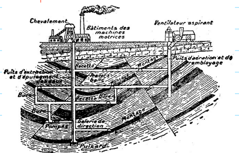
Fig. 19. — Aménagement général d'une mine ; coupe schématique.
