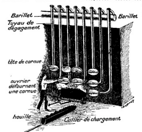
Fig. 37. — Ancien procédé de defournement et de chargement d'une corne à gaz ; emploi du crochet et de la cuiller.
